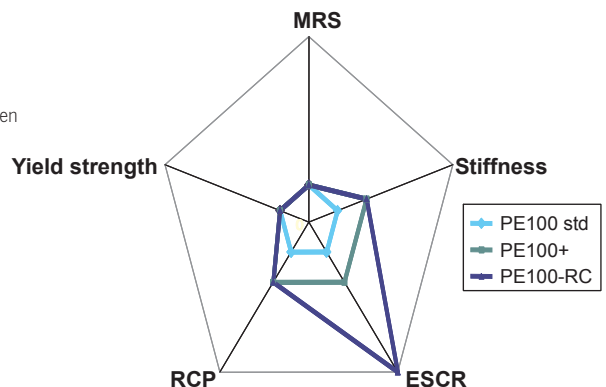
Bild 4: Vergleich maßgebender Eigenschaften von PE 100-Werkstoffqualitäten (Quelle: INEOS Polyolefins, TOTAL Petrochemicals) Fig. 4: Comparison of relevant properties of PE 100-material qualities (Source: INEOS Polyolefins, TOTAL Petrochemicals)
